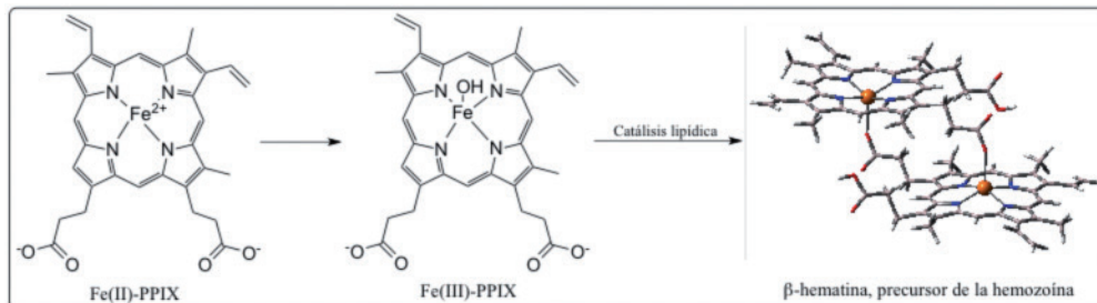
Gráfico 5.14 Mecanismo de detoxificación natural del Plasmodium mediante agregación de la hemoína a \beta -hematina, precursor de la hemozoína. Imagen molecular 3D de la \beta -hematina generada con GaussView, Version 5
