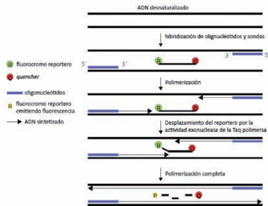
Gráfico 3.1 Esquema del mecanismo de amplificación de PCR en tiempo real utilizando sondas TaqMan para la detección del producto de la reacción
