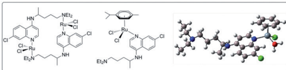
Gráfico 5.16 Complejos metal-cloroquina desarrollados por nuestro grupo de investigación con alta actividad in vitro contra cepas de Plasmodium falciparum resistentes a la cloroquina. Imagen molecular 3D del complejo rutenio-cloroquina generada con GaussView, Version 5
