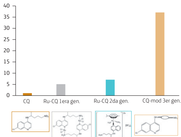
Gráfico 5.17 Evolución de nuestro diseño molecular para nuevos antimaláricos activos contra Plasmodium falciparum resistente a la cloroquina. Las actividades relativas se expresan con respecto a la cloroquina, a la cual se asigna un valor de 1. Nuestra primera generación de drogas organometálicas en 1996 logró un aumento de alrededor de tres veces en la actividad; la segunda generación, publicada en 2009, muestra un incremento por un factor cercano a cinco y resultados recientes aún no publicados elevan la actividad relativa hasta un factor de 40 en el caso de parásitos altamente resistentes
