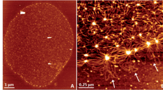
Gráfico 6.6 Red completa de DNA cinetoplástico aislado del tripanosomatideo. C. fasciculata (A). En (B), detalles del DNA cinetoplástico mostrando los agrupamientos de las moléculas de DNA formando rosetas alrededor de la periferia de las redes (flechas)
