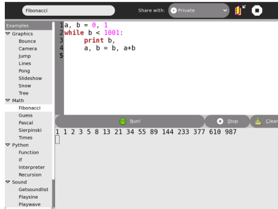
Figura B.19: Pippy : editor de código del lenguaje de programación python con ejemplos incluidos y un entorno de ejecución.
