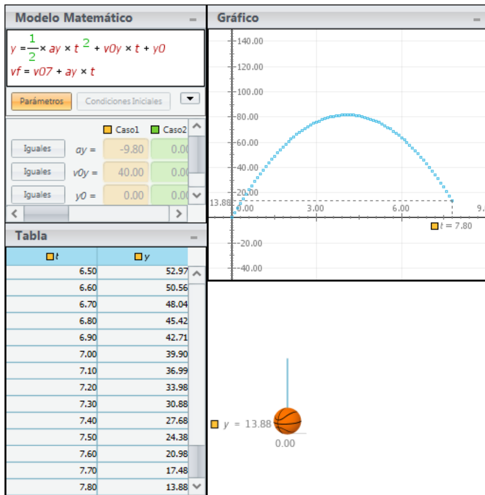
Simulación del tiro vertical de una pelota de básquet realizada con Modellus.
