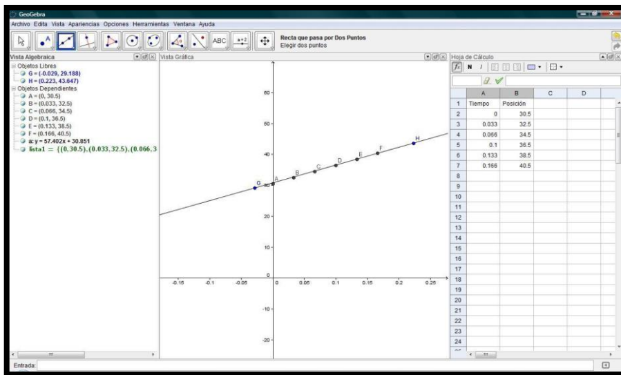
Figura 5: Análisis de los datos de posición de la bolita en función del tiempo.
