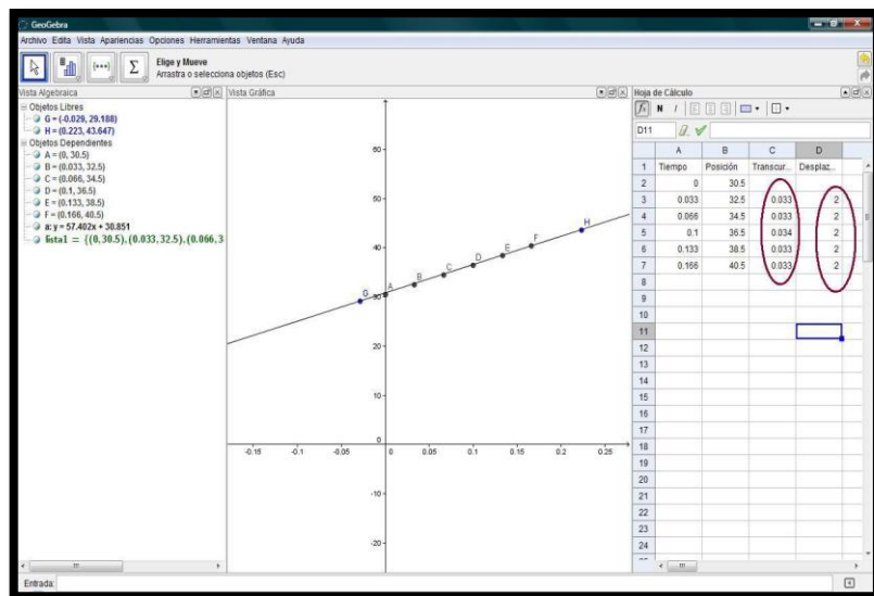
Figura 6: Análisis de datos con la planilla de cálculo de GeoGebra.
