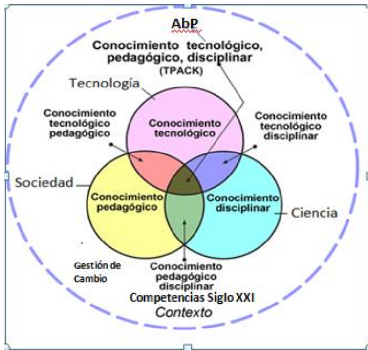
Modelo TPACK
