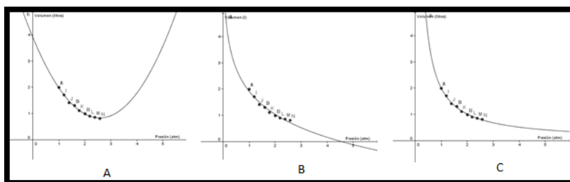
Figura 3: Gráficos de volumen en función de la presión tal como se obtienen en el programa GeoGebra. A) Conjunto de datos completos ajustados mediante una función cuadrática; B) conjunto de datos completos ajustados con una función logarítmica; C) conjunto de datos completos ajustados con una hipérbola.
